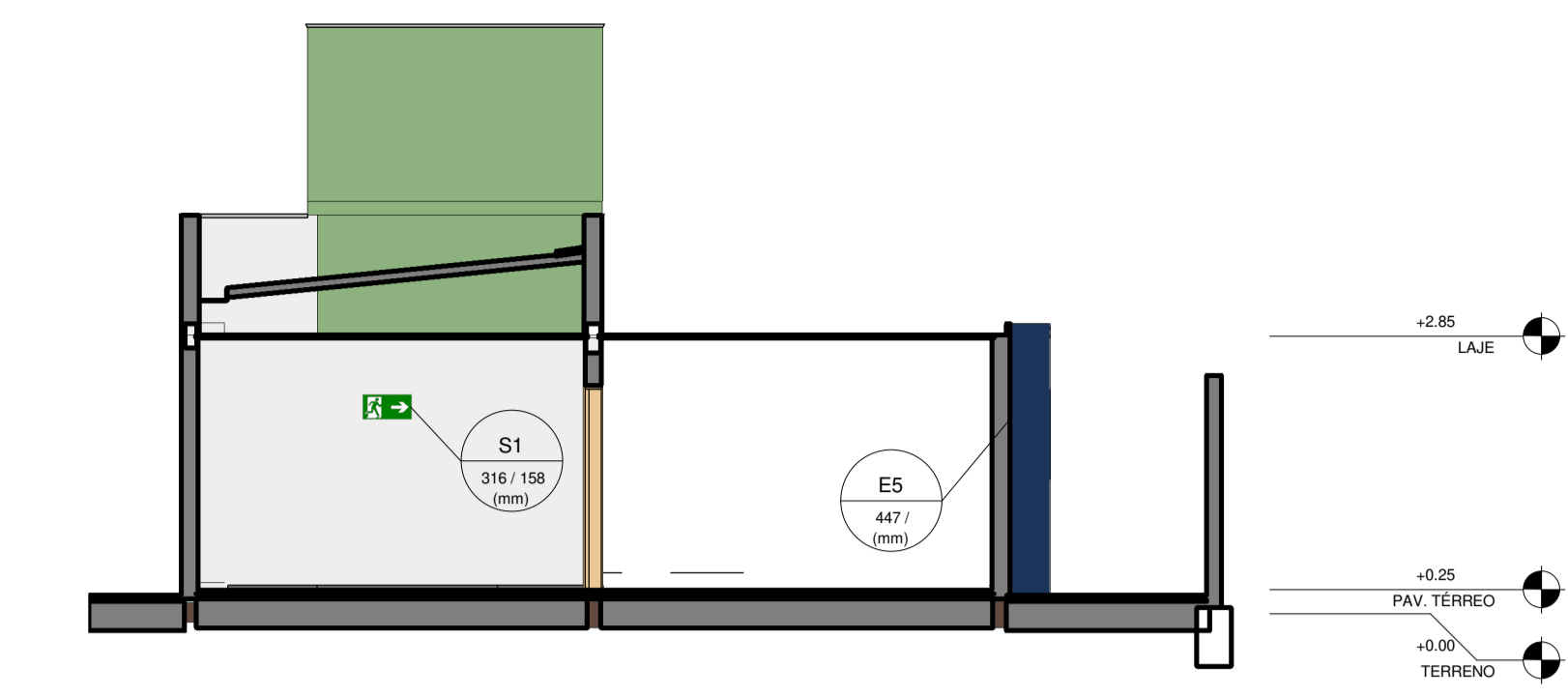
6 CORTE HH' ESCALA 1:75
