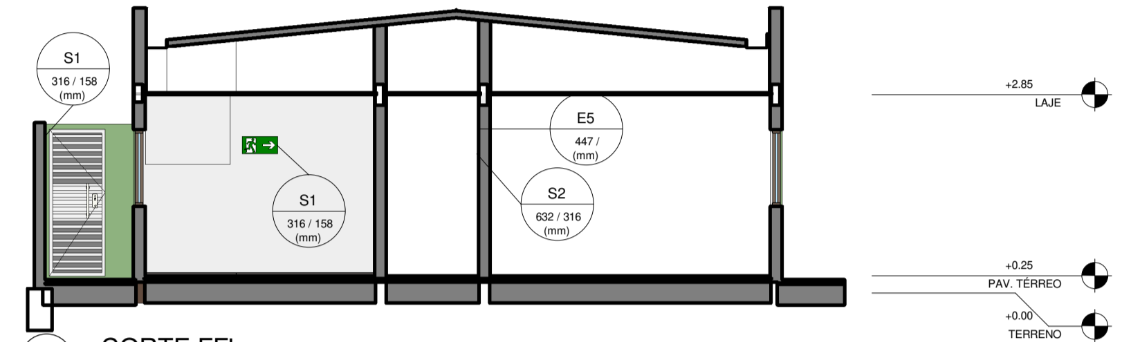
4 CORTE FF' ESCALA 1:75
