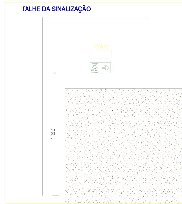
SINALIZAÇÃO DE ORIENTAÇÃO E SALVAMENTO ESCALA LIVRE
