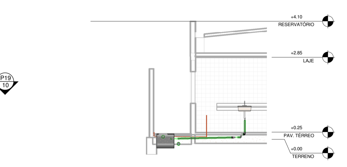
11 CORTE NN' ESCALA 1:75
