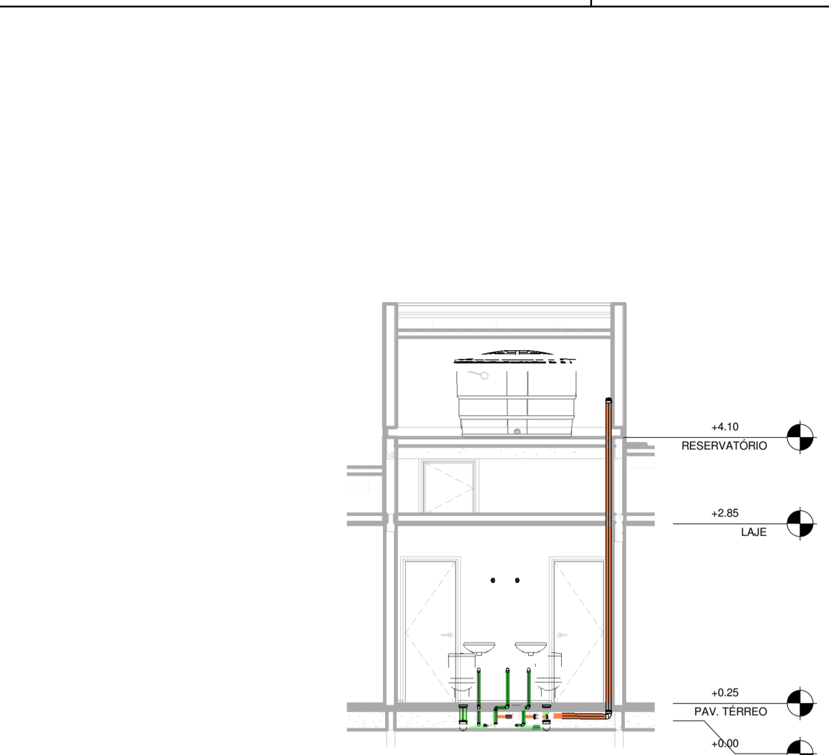
7 CORTE JJ' ESCALA 1:75
