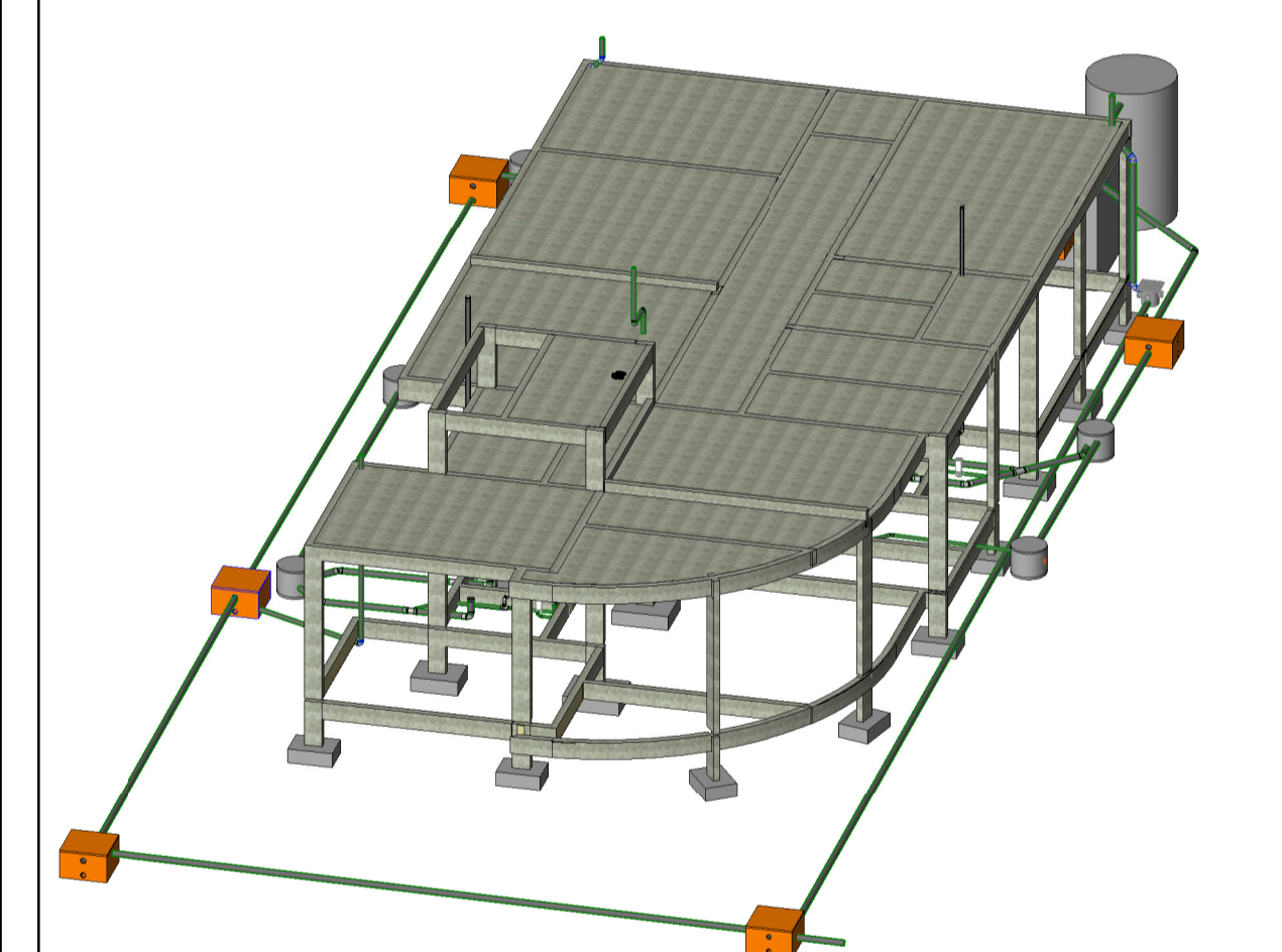
1 3D - SANITÁRIO ESCALA 1:25
