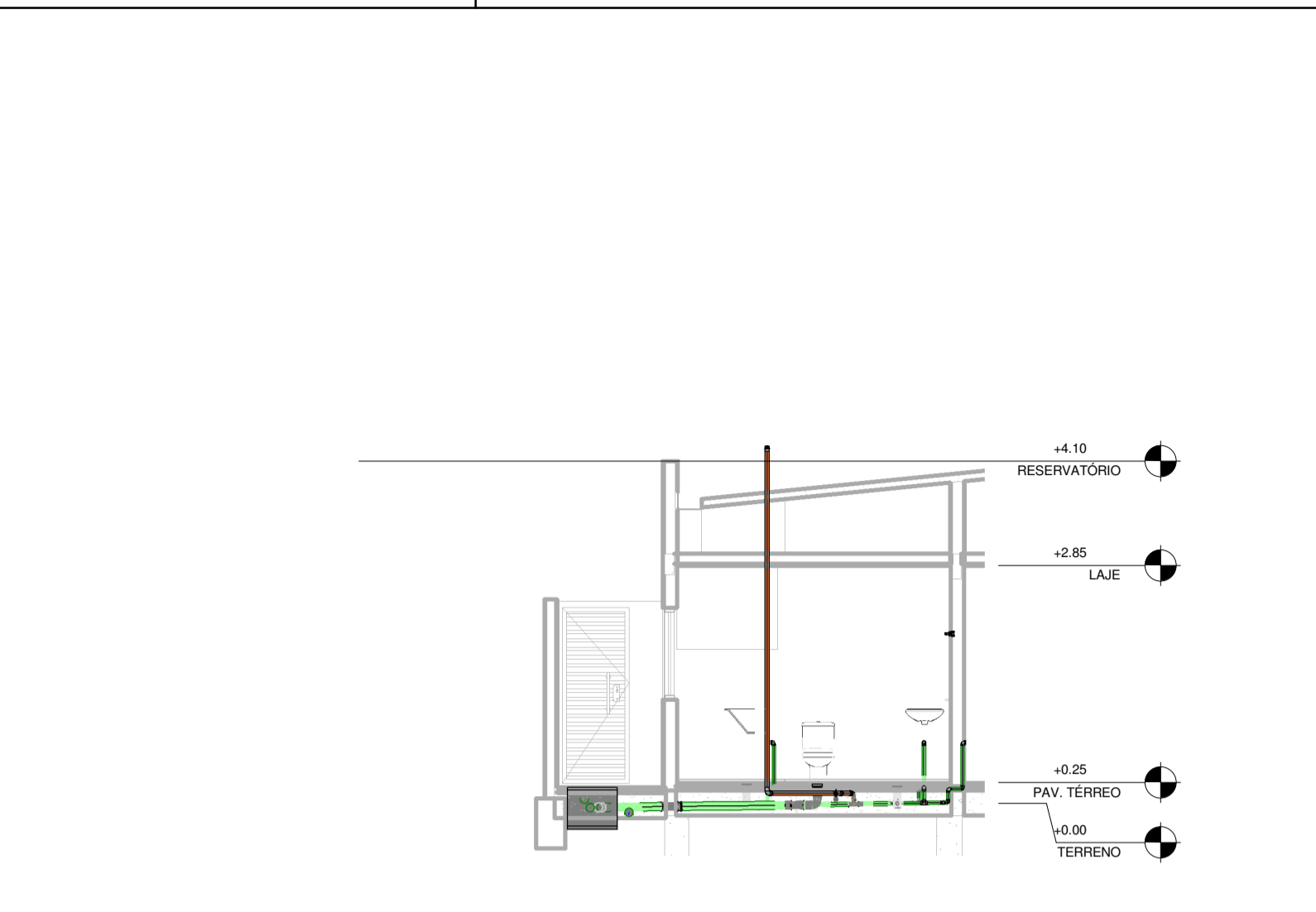
10 CORTE MM' ESCALA 1:75
